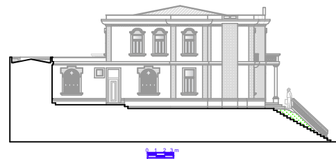
Elevation 02
