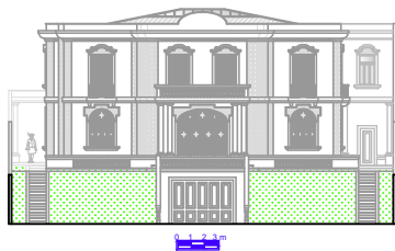
Elevation 01
